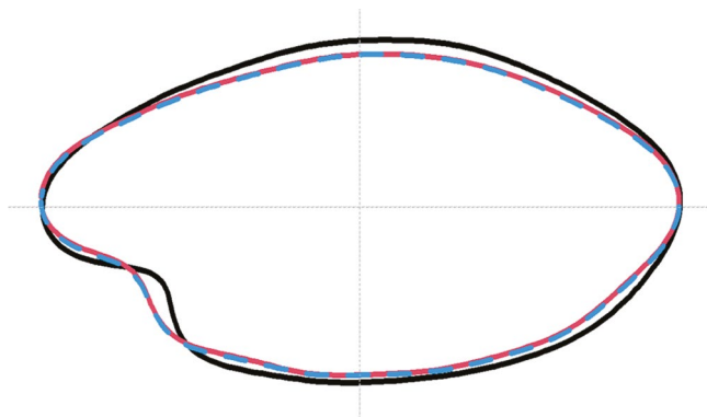
Рис. 3. Усреднённые формы отолитов азово-черноморской хамсы Engraulis encrasicolus , полученные на основе реконструкции Фурье в программе ShapeR для рыб из региона 1 (см. рис. 1): (—) — мелкие особи TL < 9 см ( n = 123 ); (—) — самки TL \geq 9 см ( n = 419 ); (—) — самцы TL \geq 9 см ( n = 402 ).
