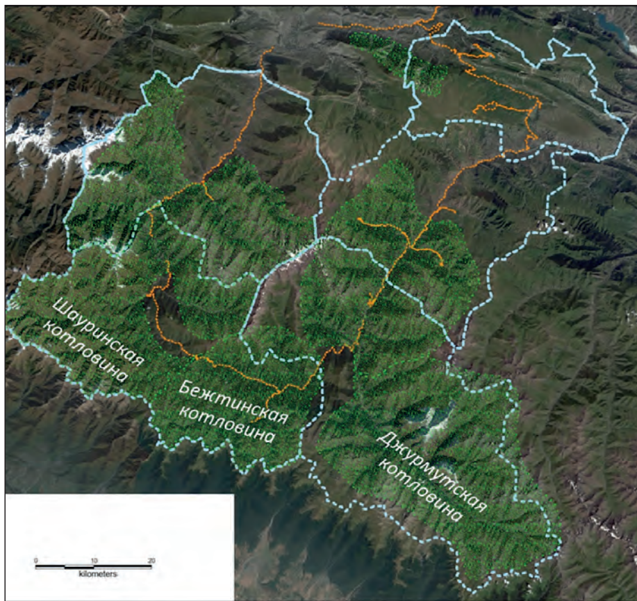
Рис. 3. Оптимальные местообитания переднеазиатского леопарда в Республике Дагестан.
