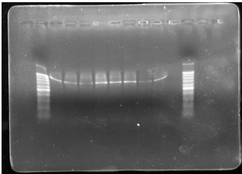
Рисунок 4. Пример подбора условий амплификации Д-петли мтДНК. В крайних лунках находится маркёр 100 п.н. Слева направо находится амплификат, полученный при разных температурах, градиент 48–58 °С, шаг изменения температуры приблизительно 1.2 °С градуса, 35 циклов ПЦР. Амплификация проводилась с праймерами Trpo2 и NH20, полимеразы Screen Mix (Евроген).
